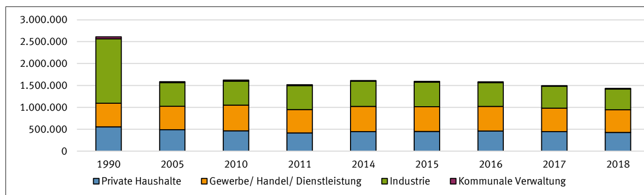
Abb. 6.3 CO 2 -Emissionen nach Verursachern in Mainz seit 1990 (in Tonnen/Jahr)*
