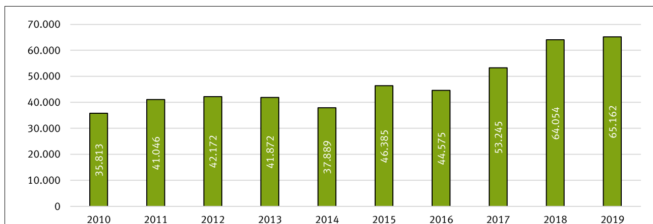
Abb. 6.1 Eingespeister Strom aus erneuerbarer Energie in MWh in Mainz seit 2010
