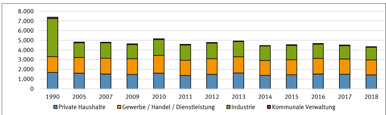
Abb. 6.2 Endenergieverbrauch nach Verbraucher:innen in Mainz seit 1990 (in GWh/a)*
